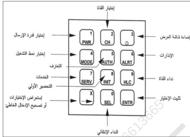
الشكل رقم (128) لوحة الأزرار
