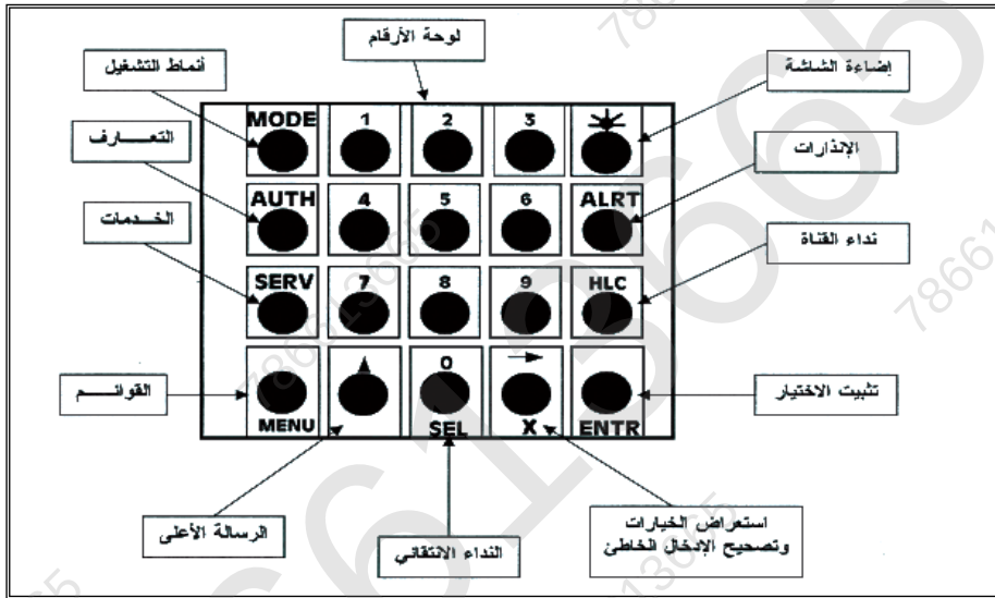
الشكل رقم (124) لوحة أزرار إدخال المعلومات
