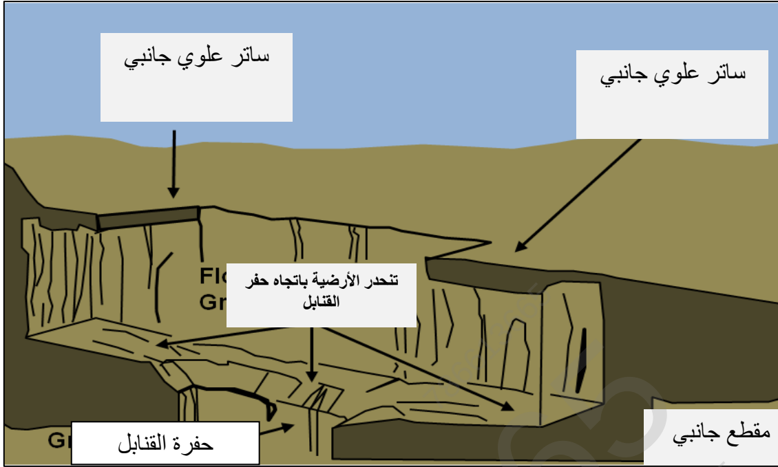
الشكل رقم (137) ساتر علوي جانبي
