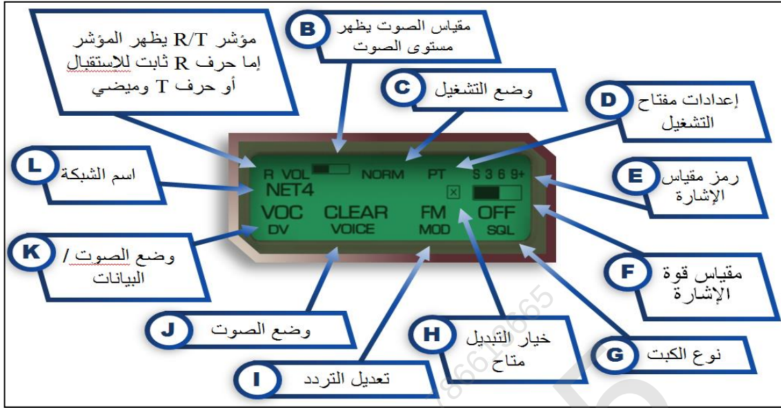
الشكل رقم (112) شاشة عرض جهاز هاريس RF-5800V-HH المحمول باليد (1)
