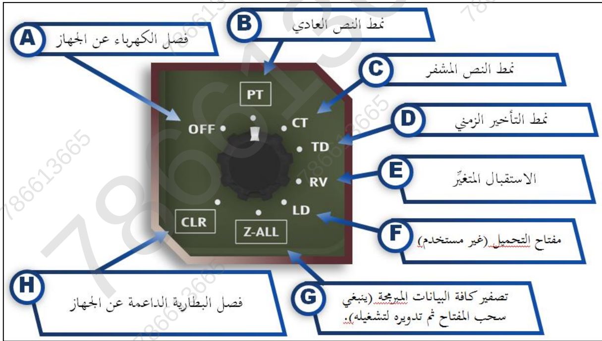
الشكل رقم (105) إختيار مفتاح التشغيل
