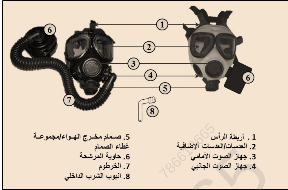
الشكل رقم (144) قناع الوقاية وأجزائه الرئيسية
