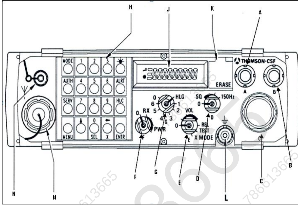
الشكل رقم (119) اللوحة الأمامية لجهاز TRC 9200
