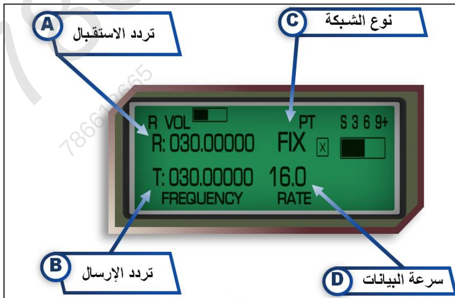
الشكل رقم (108) شاشة العرض لنمط التشغيل الاعتيادي-2
